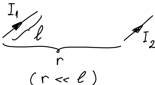
Фигура 3: Сила на Ампер
