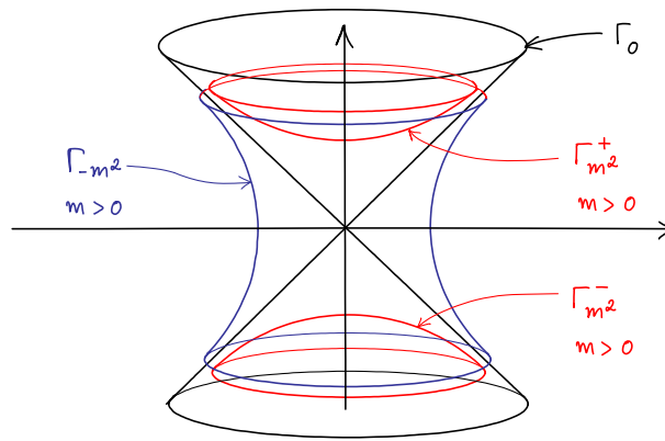
Фигура 12: Хиперболоиди. Във връзка с релативистката динамика, параметърът \pm a > 0 е положен като a = m^2 и новия параметър m ще има смисъл на релативистка маса.
