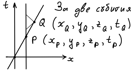
Фигура 9: Релативистки интервал в общия случай на инерциални наблюдатели.
