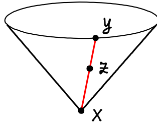
Фигура 6: Мировата линия на светлинен сигнал е образуваща права на светлинен конус
