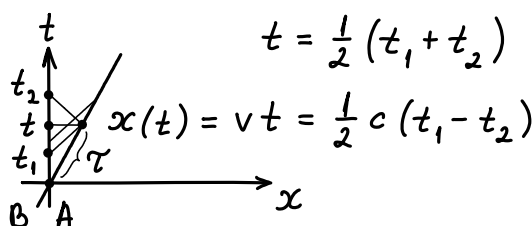
Фигура 7: Пресмятане на коефициента на Доплер
