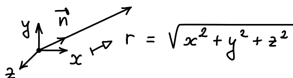
Фигура 8: При движение вместо по оста x по произволна ос определена от вектор \mathbf{n} ролята на координатата x се заменя с разстоянието r по оста \mathbf{n} .
