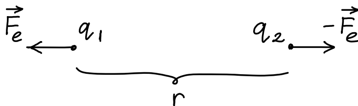
Фигура 2: Електростатични сили между два едноименни (еднакви по знак) точкови заряди
