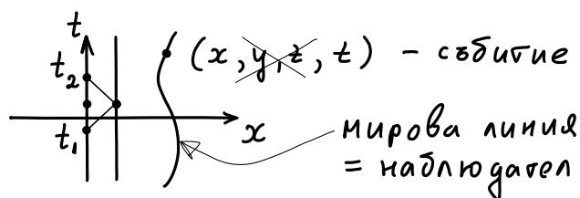
Фигура 5: Пространство времева диаграма изобразяваща радио-локационния метод. Мировата линия на наблюдателя A съвпада с времевата ос t . Светлинните импулси също имат мирови линии, които са двете наклонени отсечки излизащи от оста t . За простота на чертежа сме избрали движението да се извършва по оста x , поради което останалите координати y и z на фигурата са равни на нула. На диаграмата сме начертали освен мировата линия на измервания наблюдател, който е избран неподвижен спрямо A , също и една мирова линия на произволно движещ се наблюдател.
