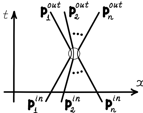
Фигура 9: Закон за запазване на импулса при сблъсък на n материални точки (тела): точки с начални (нерелативистки) импулси \mathbf{p}_1^{in}, \dots, \mathbf{p}_n^{in} , взаимодействат в малка област на пространство-времето, което можем да си мислим в пределния случай, като моментен точков сблъсък. След сблъсъка те получават импулси съответно равни на, \mathbf{p}_1^{out}, \dots, \mathbf{p}_n^{out} . Според закона за запазване на импулса: \mathbf{p}_1^{in} + \dots + \mathbf{p}_n^{in} = \mathbf{p}_1^{out} + \dots + \mathbf{p}_n^{out} .
