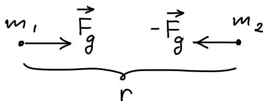
Фигура 1: Гравитационно привличане между две материални точки
