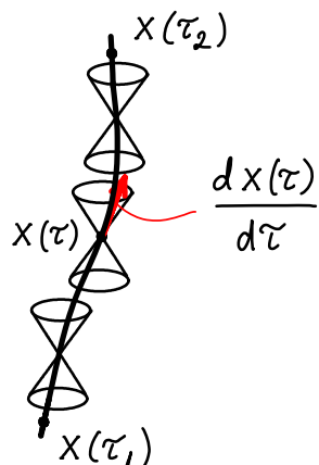
Фигура 2: Време-подобна мирова линия
