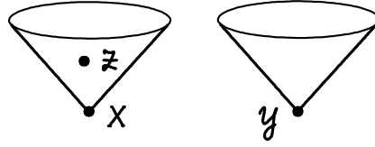
Фигура 5: Пространствено-подобие не е транзитивно
