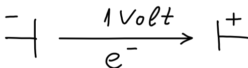
Фигура 4: Електронволт е енергията, която придобива (или губи) електрон при преминаване през електричен потенциал от 1 волт (Volt)
