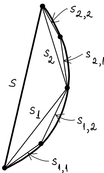
Фигура 3: Псевдо-евклидово неравенство на триъгълника
