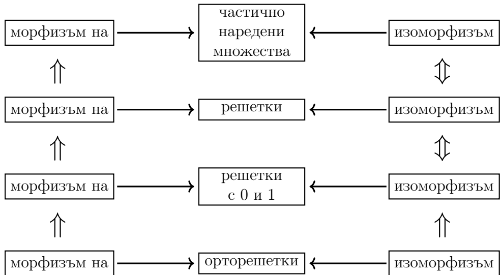
фиг. 32: Взаимовръзка между различните категории морфизми
