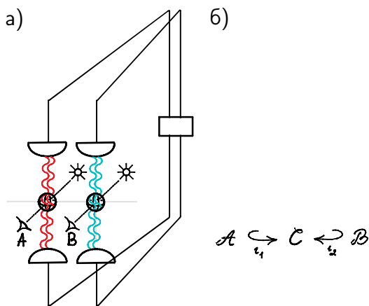
фиг. 56: Начална постановка на съставна система от два квантови бита:
