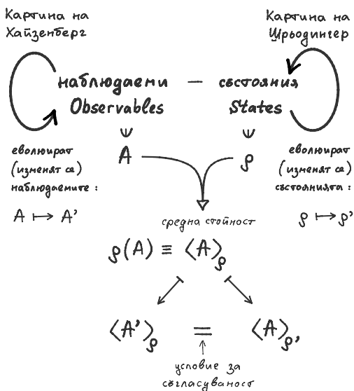
фиг. 61: Двете картини на квантовите трансформации.
