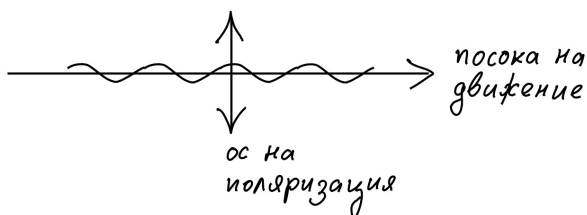
фиг. 2: Линейно поляризираната електромагнитна вълна е класическия “предобраз” на линейно поляризиания фотон.
