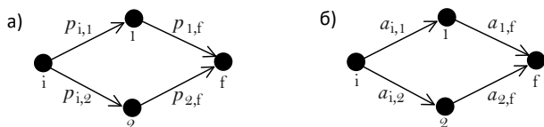
фиг. 15: Преход между две състояния i \rightarrow f през две алтернативни състояния 1 и 2 - а) класически; и б)
