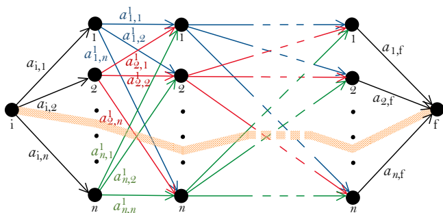
фиг. 16: Преход между състояния i \rightarrow f на няколко стъпки през алтернативни междинни състояния. В определени условия, наречени във физиката “класическа граница” амплитудите на повечето пътища се погасяват взаимно и остава един доминиращ път - оцветения с плътна оранжева линия - това е “класическата траектория” на системата.
