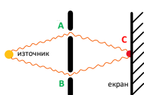
фиг. 14: Нарушение на дистрибутивността
