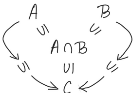
фиг. 7: Сечение в частично наредено множество
