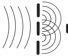
фиг. 10: Общата картина на локалното разпределение на преминалите частици изглежда като картина на интерференция на вълни. Да напомним, че при интерференцията имаме наред с усилващото събиране на вълните също и взаимно погасяване в определени точки.
