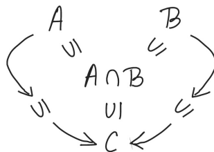
фиг. 7: Сечение в частично наредено множество
