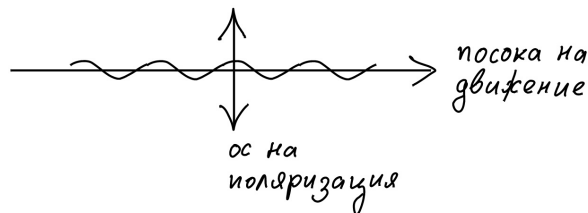
фиг. 2: Линейно поляризираната електромагнитна вълна е класическия “предобраз” на линейно поляризирания фотон.
