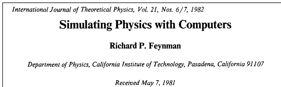
фиг. 24: Статията на Файнман от 1982 - една от първите, в които се споменава за ‘квантов компютър’
