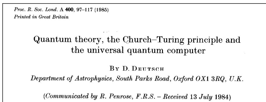
фиг. 25: Статията на Дойч от 1986 - една от първите, в които се въвежда концепцията за квантови изчисления
