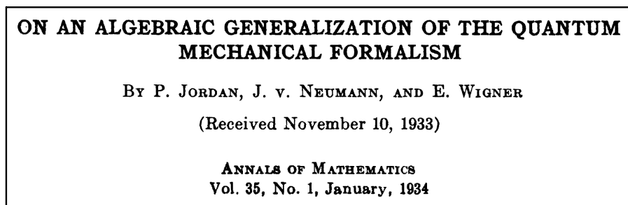
фиг. 21: Завършващата статия на алгебричния подход
