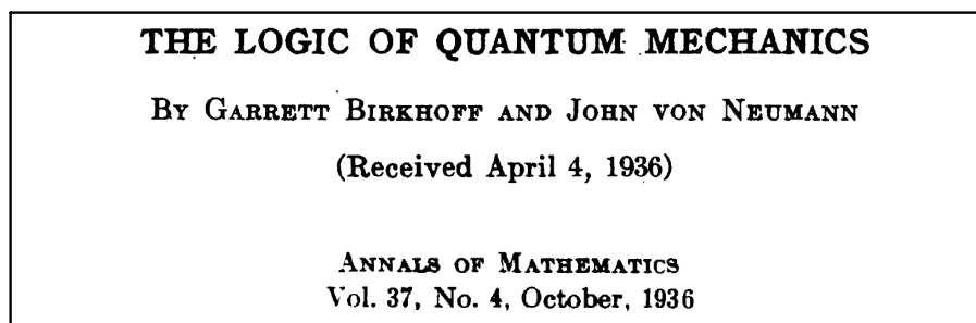
фиг. 23: Основополагащата статия на квантово-логическия подход
