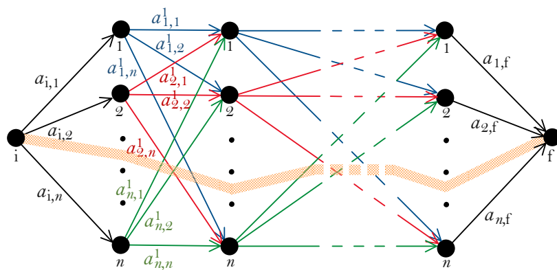
фиг. 16: Преход между състояния i \rightarrow f на няколко стъпки през алтернативни междинни състояния. В определени условия, наречени във физиката “класическа граница” амплитудите на повечето пътища се погасяват взаимно и остава един доминиращ път – оцветения с плътна оранжева линия – това е “класическата траектория” на системата.
